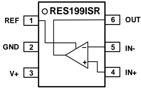
SC70-6
